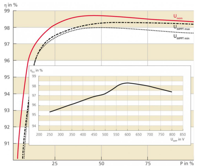
Wirkungsgradverlauf und Vergleich der MPPT-Spannung beim StecaGrid 5003
