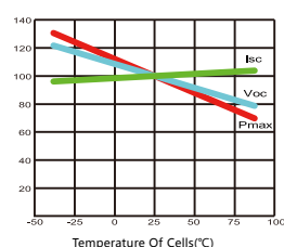
LP182*182-M-60-MH-440W
