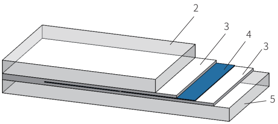
Bifacial-Doppelglasmodul (Rahmenlos)
