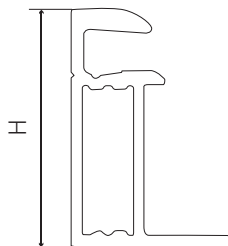
Aluminiumrahmenhöhe (H)
