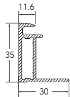
Rahmenquerschnitt
