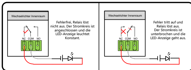
Abb. 5-6 Öffnerkontakt
