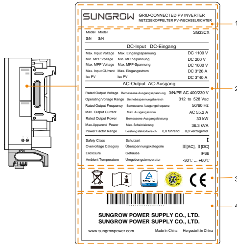
Abb. 3-1 Typenschild
