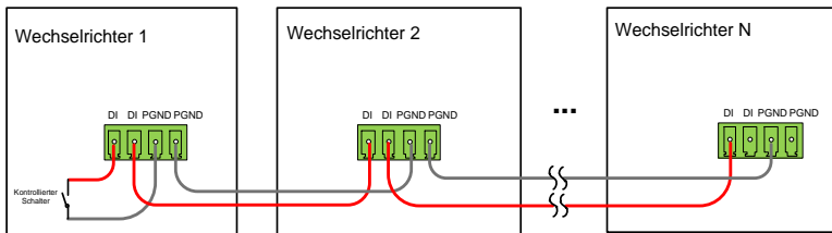
Abb. 5-8 Daisy-Chain-Topologie
