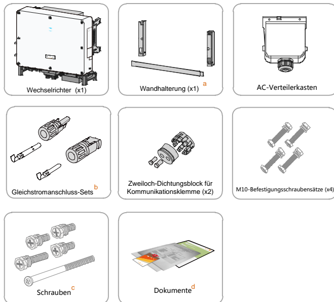
Abb. 3-2 Lieferumfang
