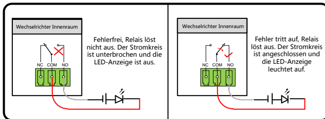
Abb. 5-5 Schließkontakt
