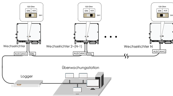
Abb. 5-4 Status Abschlusswiderstände
