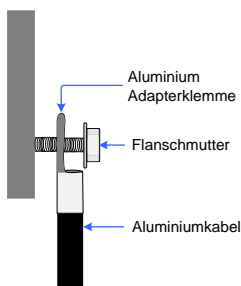
Abb. 5-3 Anschlussreihenfolge der Aluminium-Kabelklemmen
