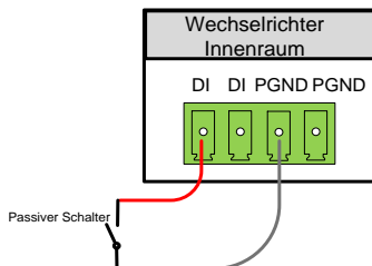
Fig. 5-8 Lokaler Stopp-Kontakt
