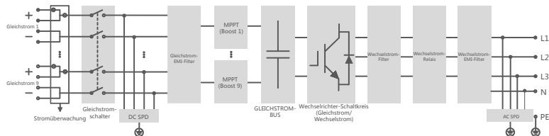
Fig. 2-6 Schaltplan
