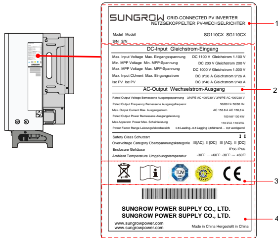
Fig. 3-1 Typenschild
