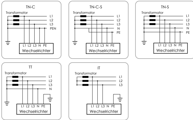
Fig. 2-2 Netztypen
