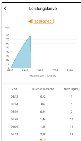
Fig. 7-10 Leistungsablauf
