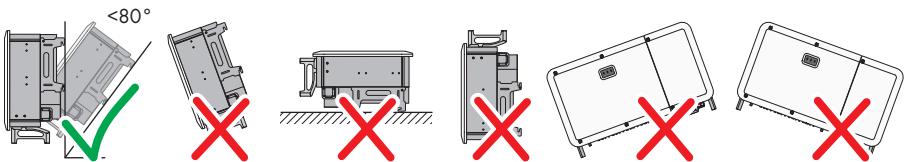
Abbildung 3: Zulässige und unzulässige Montagepositionen
