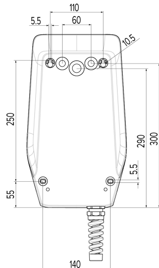
Fig. 6: Borrmått [mm]
