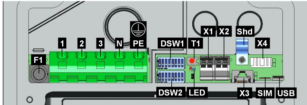
Abb. 7-15: Anschlussübersicht
