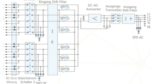
Schaltplan
