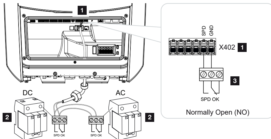
Abb. 6: Überspannungsschutz (SPD) als Schließler
