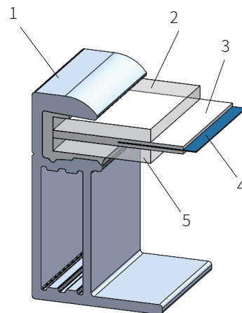
Bifacial-Doppelglasmodul (Mit Rahmen)
