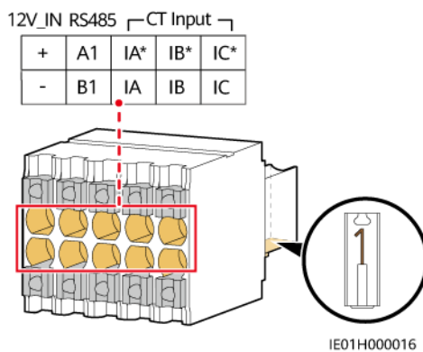
Abbildung 5-5 10-poliger Stecker
