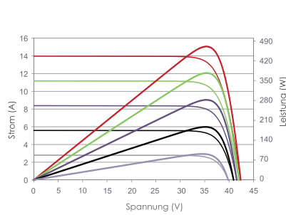
Strom-Spannungs- und Leistungs-Spannungs-Kennlinien (430W)
