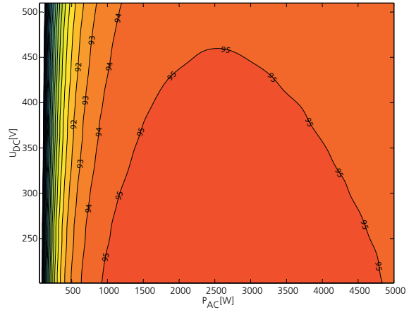
3D-Wirkungsgraddiagramm Powador 6002
