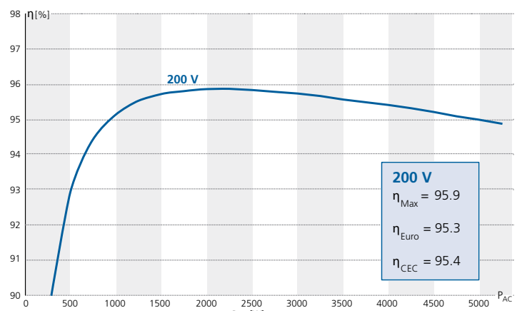
Wirkungsgradkennlinie Powador 6002
