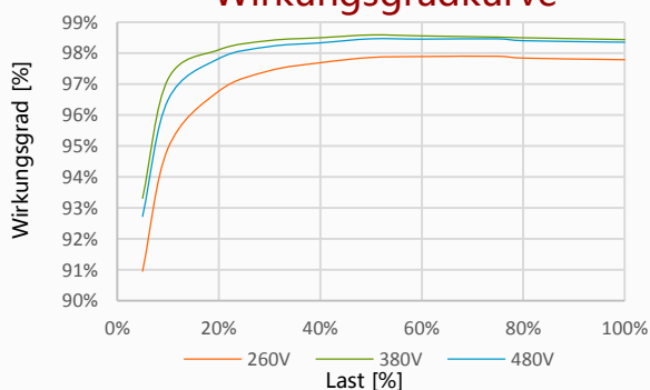
Wirkungsgradkurve
