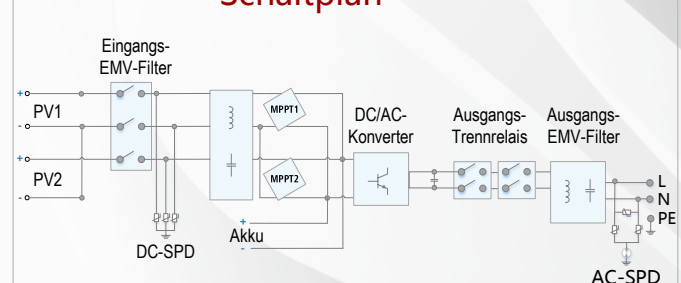
Schaltplan
