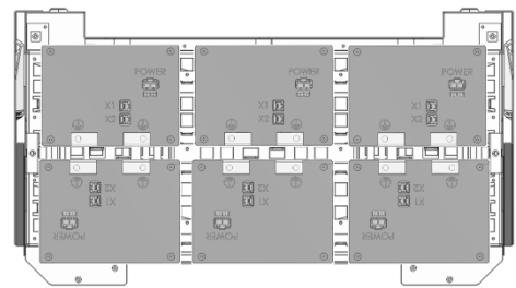
Mit 6 Helios Batteriemodulen
