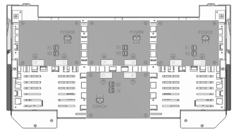
Mit 4 Helios Batteriemodulen
