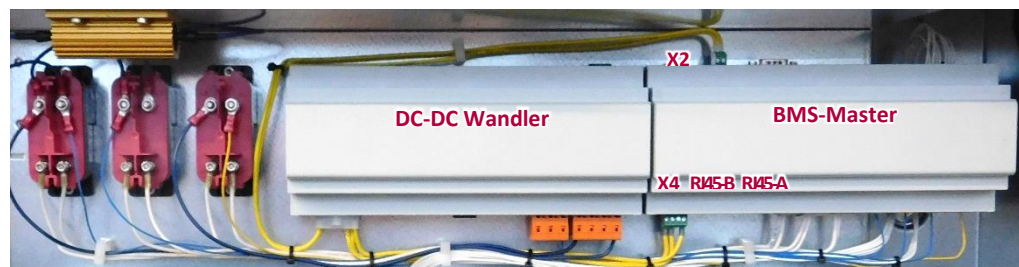
Abbildung 9: Anordnung BMS-Master, DC-DC Wandler, Relais und Vorladewiderstand
