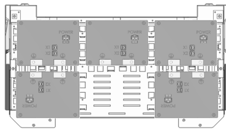
Mit 5 Helios Batteriemodulen
