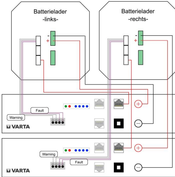
Abbildung 17: Verbindungen – Ausbaustufe element 9/12
