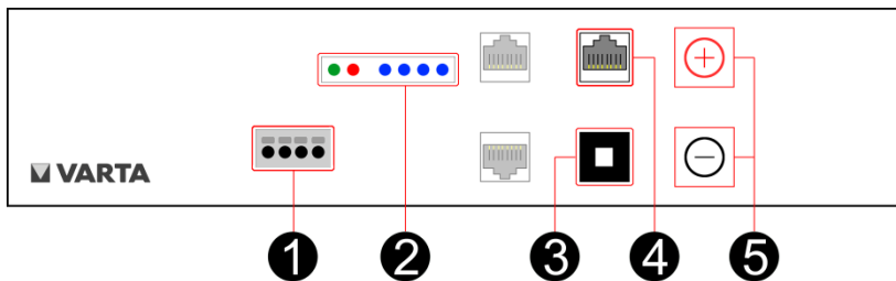
Abbildung 29: Batteriemodul
