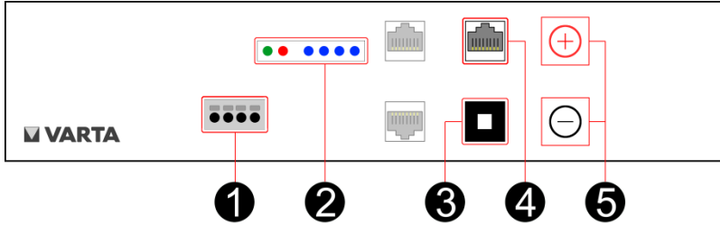
Abbildung 13: VARTA element Batteriemodul
