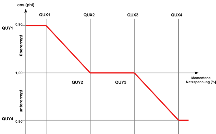
Abbildung 22: Q(U)-Kennlinie
