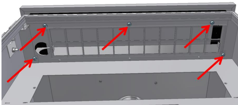
Abbildung 31: Schrauben Schrankdeckel – (vorne-unten)
