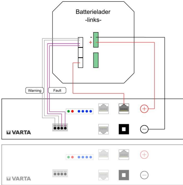
Abbildung 16: Verbindungen - Ausbaustufe element 6
