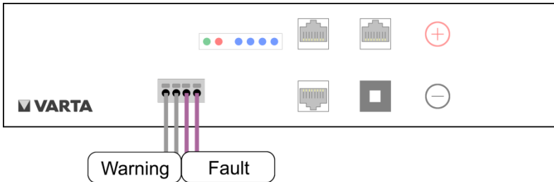
Abbildung 14: Klemmverbindungen Batteriemodul (DRY-contact)
