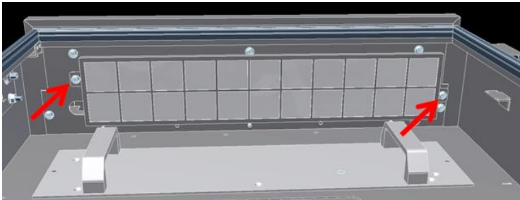
Abbildung 30: Luftfilter ausbauen (von vorne-unten)
