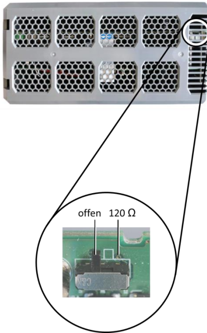
Abbildung 28: Abschlusswiderstand einstellen
