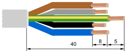
Abbildung 6: Kabel abisolieren
