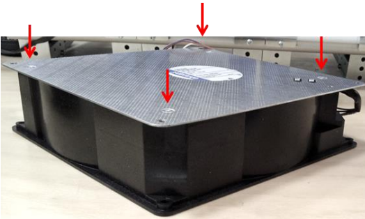
Abbildung 34: Plastikgehäuse entfernen
