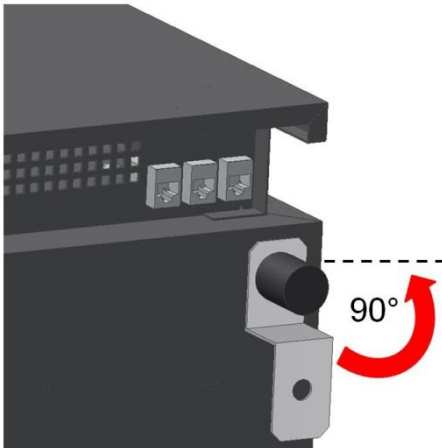
Abbildung 11: Wandbefestigung VARTA element
