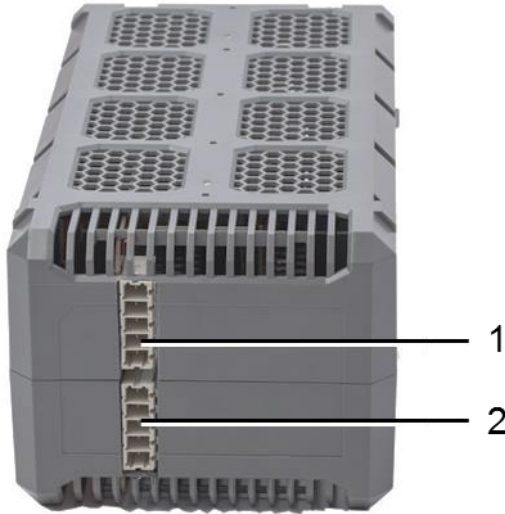
Abbildung 27: Batterielader – Rückseite
